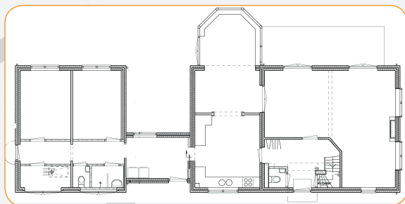
Bestaande situatie begane grond
