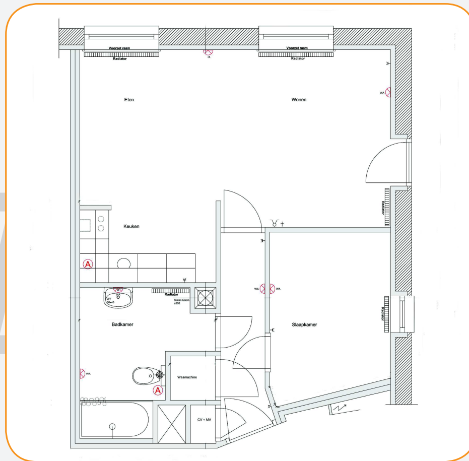
Bestaande situatie begane grond
